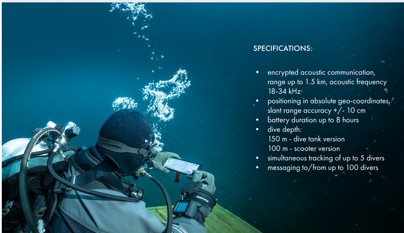
Diver modem unit
